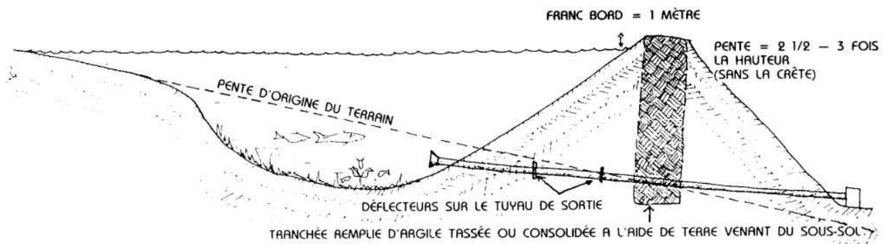
FIG. 7.2 : UN BARRAGE CLASSIQUE (D'APRES YEOMANS 2 ) SECTION
