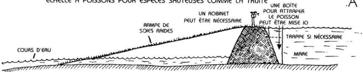
ÉCHELLE A POISSONS POUR ESPÈCES SAUTEUSES COMME LA TRUITE
