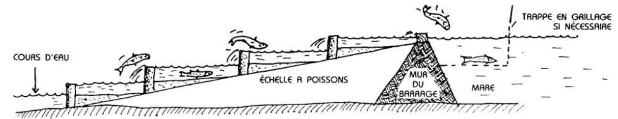
ÉCHELLE A POISSONS POUR ESPÈCES SAUTEUSES COMME LA TRUITE
