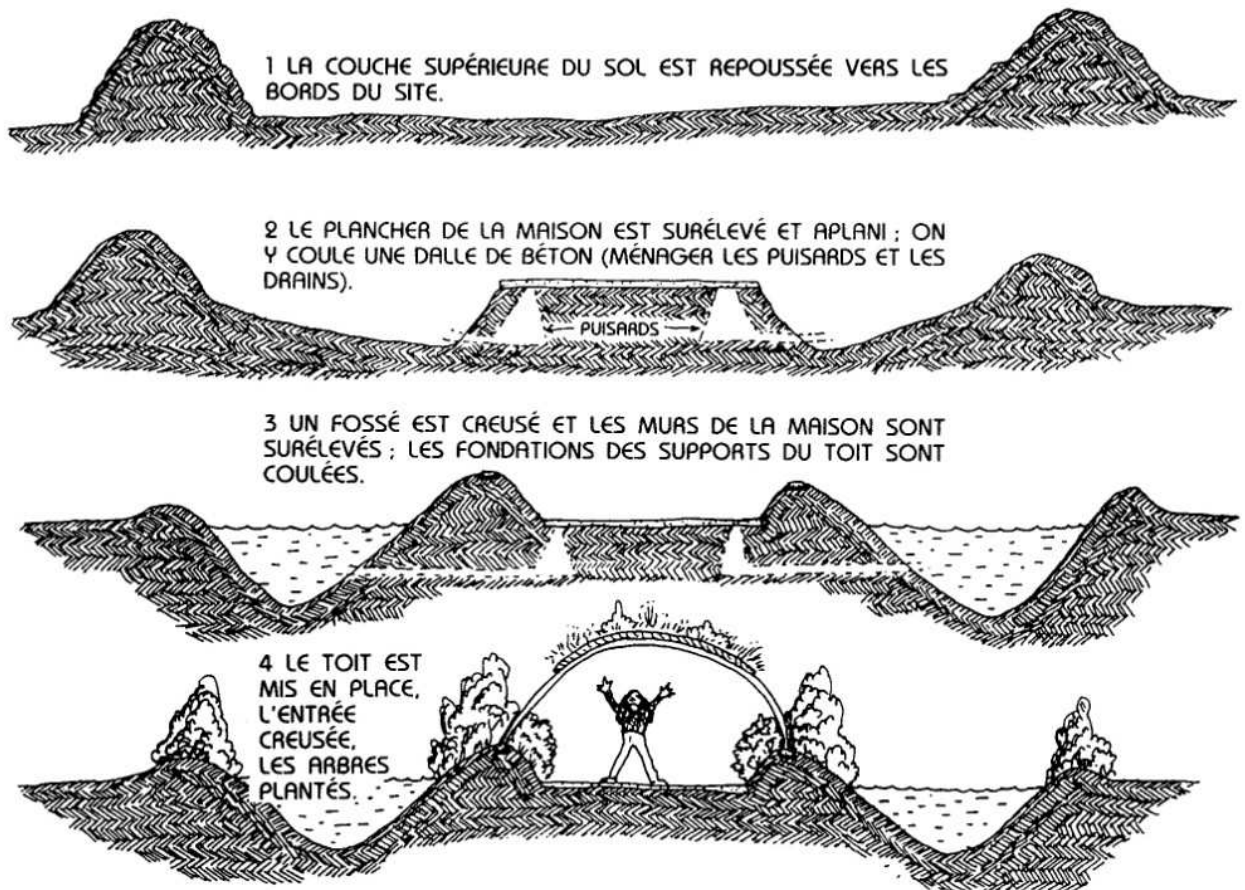
FIG. 6.5: STADES DE OONSTRUCTION D'UNE MAISON EN TERRE.
