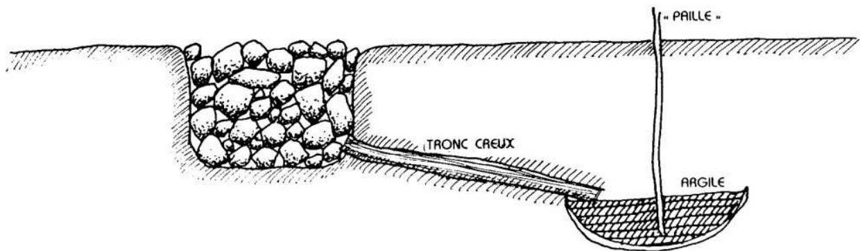
FIG. 5.19: CONDENSATEUR LOCAL UTILISÉ EN AUSTRALIE OCCIDENTALE (DONNÉES DE PHILIP GALL).
