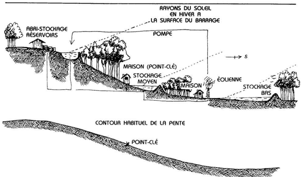
FIG. 2.7 : EMLACEMENT IDEAL DES ELEMENTS EN RELATION AVEC LA PENTE.
