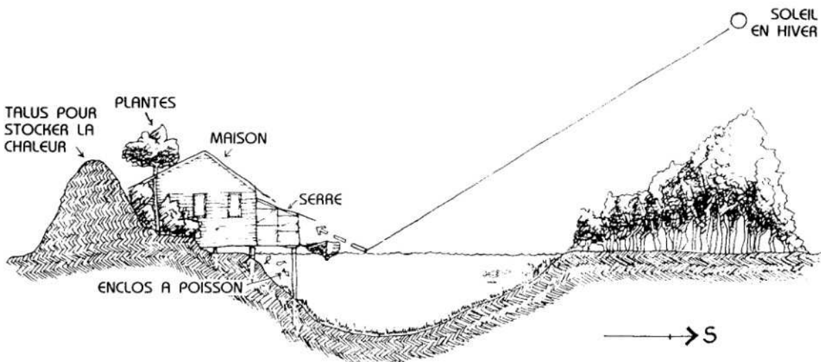
FIG. 2.9 : DES BARRAGES UTILISÉS POUR RÉFLÉCHIR LE SOLEIL EN HIVER ACCROISSENT LE MATIN, LE SOIR ET EN HIVER LA CHALEUR QUE REÇOIT LA SERRE EXPOSÉE. AU MIDI. LES PLANTES QUI S'Y TROUVENT EN BÉNÉFICIENT.
