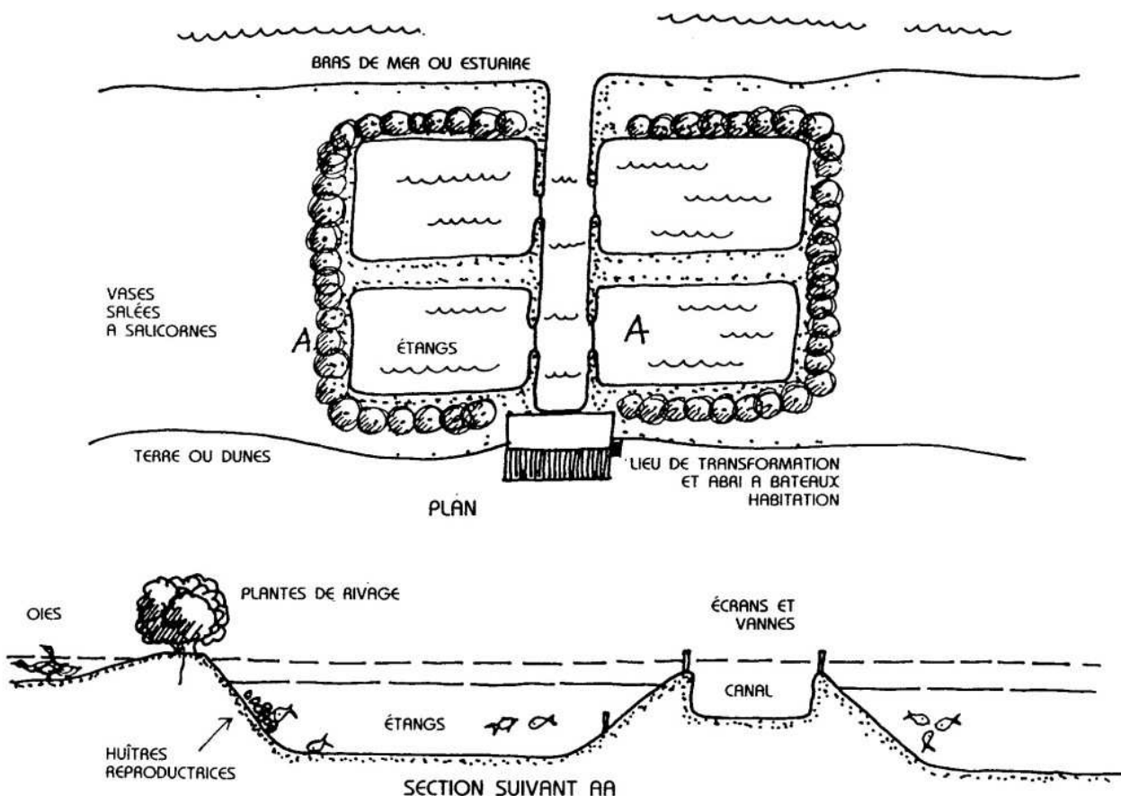
FIG. 7.24: PLAN ET SECTION D'ÉTANGS A MARÉE.
