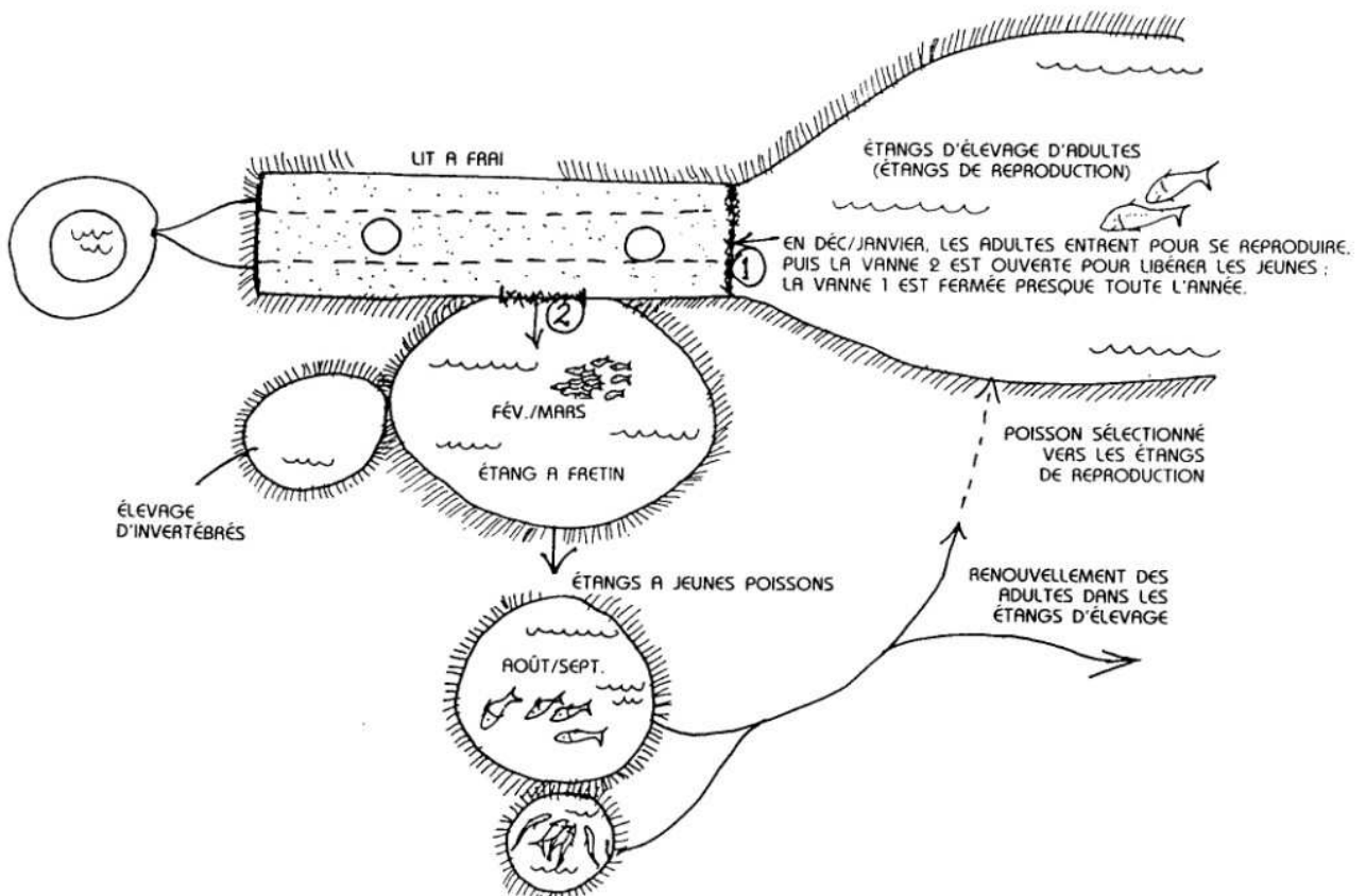
FIG. 7.22: SYSTÈME D'ÉTANG SCHÉMATISÉ (TRUITE).
