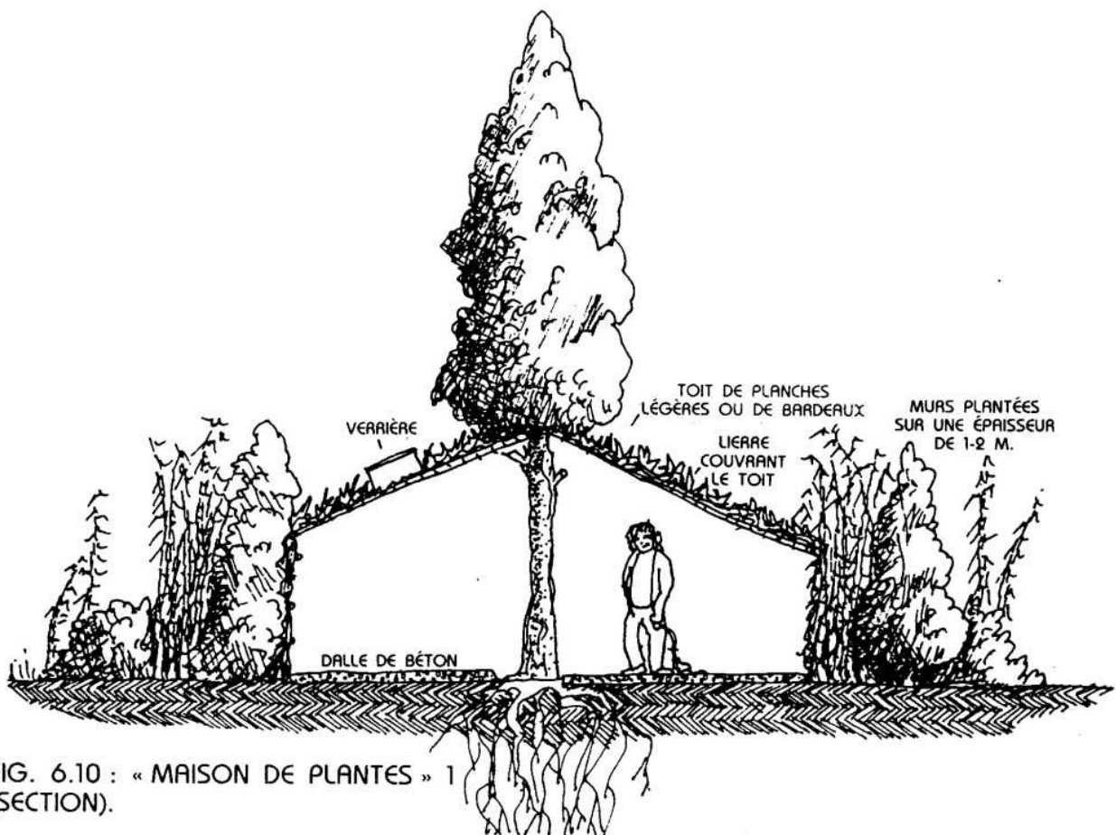
FIG. : 6.10: MAISON DE PLANTES » 1 (SECTION).
