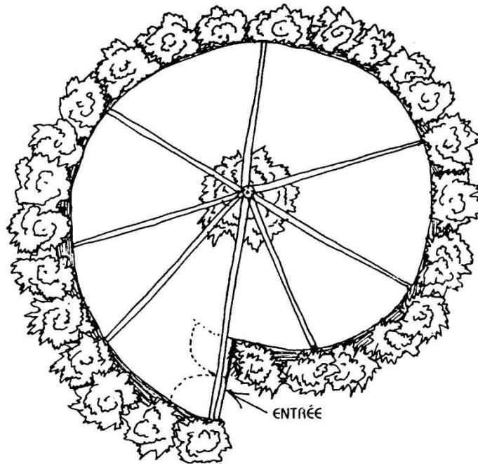
FIG. 6.9 : « MAISON DE PLANTES » 1 (PLAN) DALLE DE BÉTON AU SOL, SPIRALE DE BAMBOU OU DE PEUPLIER, PILIER CENTRAL CONSTITUTE PAR UN ARBRE EXISTANT. LES MURS SONT TISSÉS ET COUVEATS DE LIERRE JUSQU'AU TOIT. O'EST UN ABRI BON MAROHÉ POUR LE BÉTAIL.
