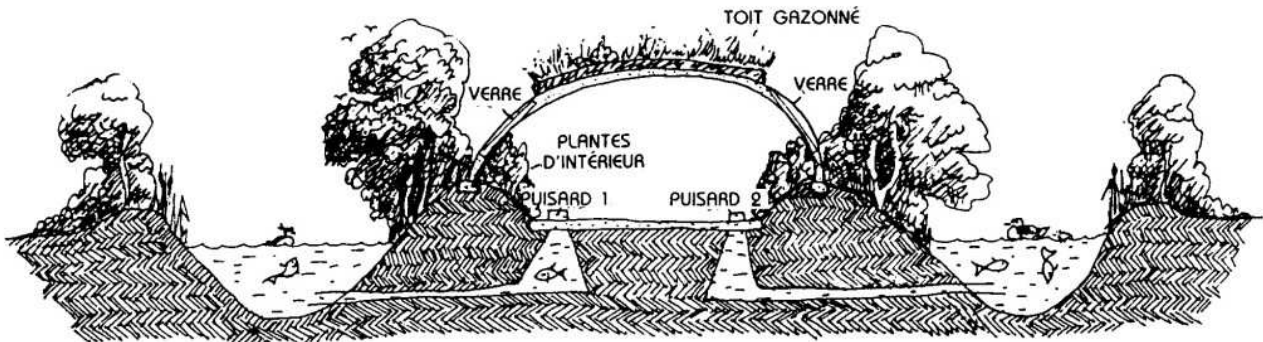
FIG. 6.6 : SECTION D'UNE MAISON EN TERRE — DES DIVISIONS LÉGÈRES PEUVENT ÊTRE ÉTABLIES A L'INTÉRIEUR. LE MUR SUD EST EN VERRE, LE MUR NORD EST EN TERRE, SANS OUVERTURE.
