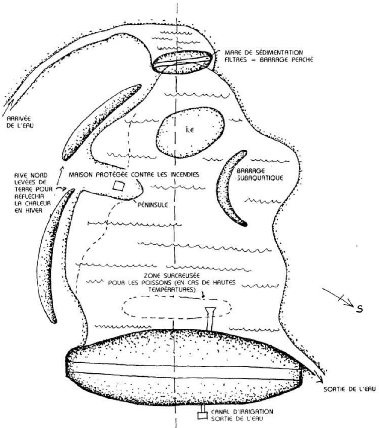
FIG. 7.3 : « COMPLICATIONS » POSSIBLES A PARTIR D'UN BARRAGE CLASSIQUE POUR ETABLIR UNE PERMACULTURE
