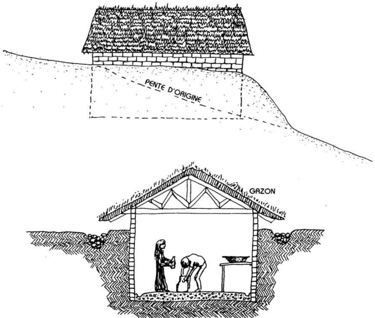
FIG. 6.8 : LAITERIE DE CAMPAGNE TRADITIONNELLE, TAILLÉE DANS LA TERRE ; LES MUAS SONT MAÇONNÉS ET LE TOIT AECOUVERT DE GAZON, LE PLANCHER EST FAIT DE TERRE BATTUE, OU BÉTONNÉ. LES AVANT-TOITS SE TERMINENT AU-DESSUS D'UN DRAIN. LA FRAÎCHEUR EST GARANTIE QUEL QUE SOIT LE TEMPS.
