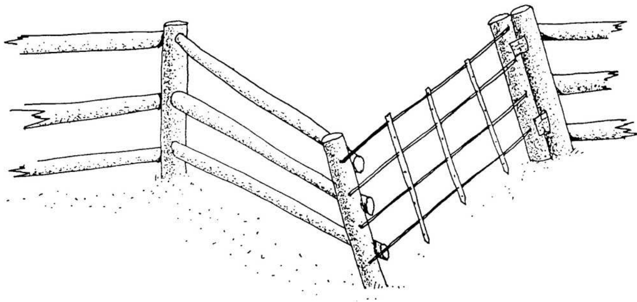
FIG. 5.23: DÉTAIL DE LA PORTE DE L'ENCLOS-PIÈGE. LES POTEAUX INCLINÉS FONT QUE LA PORTE D'ACIER RETOMBE ET SE FERME APRÈS QUE LES BOVINS ET LES CHEVAUX L'ONT OUVERTE POUR ACCÉDER A L'EAU (L'INCLINAISON EST EXAGÉRÉE ICI). D'APRÈS LE PIÈGE DE WARRENS CREEK.
