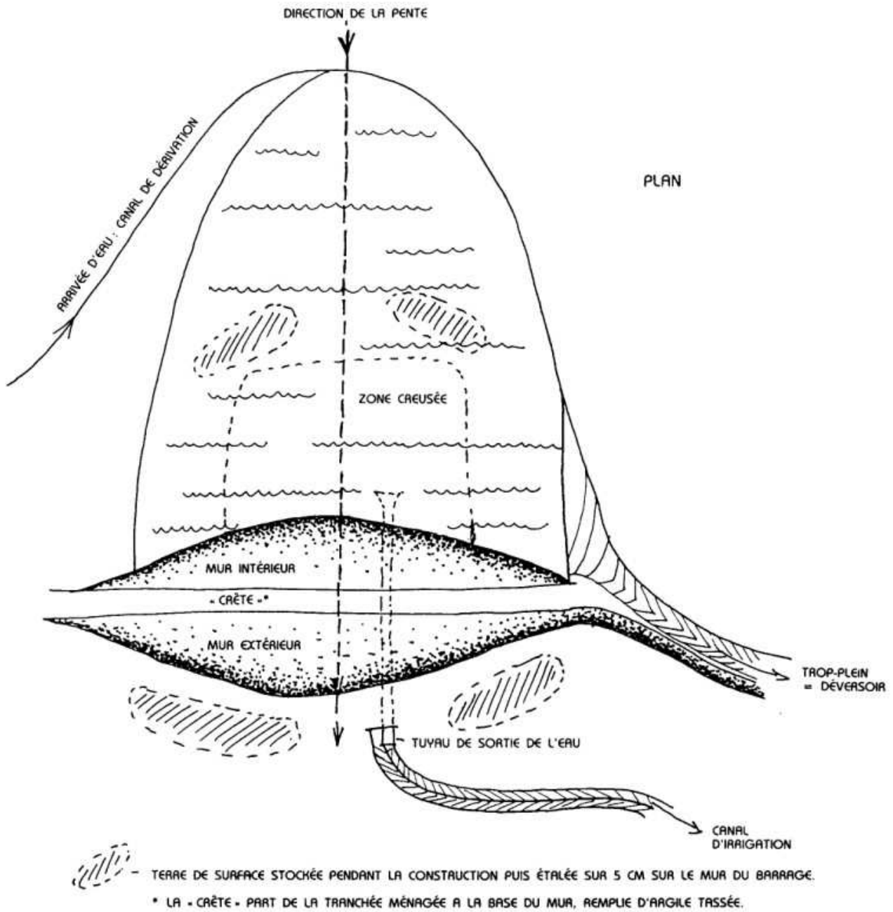
FIG. 7.1 : UN BARRAGE CLASSIQUE (D'APRES YEOMANS 2 )
