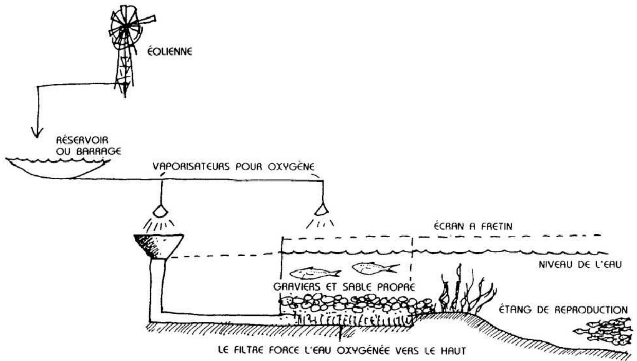
FIG. 7.21: FRAI SUR GRAVIERES POUR ESPÈCES OOMME LES TRUITES EN ÉTANG D'EAU STAGNANTE.
