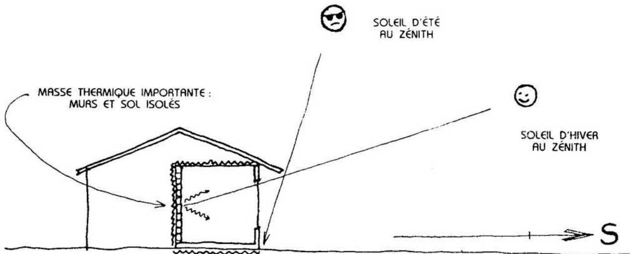
FIG. 6.21 : RELATIONS ENTRE SOLEIL, FENÊTRE ET AVANT-TOIT.
