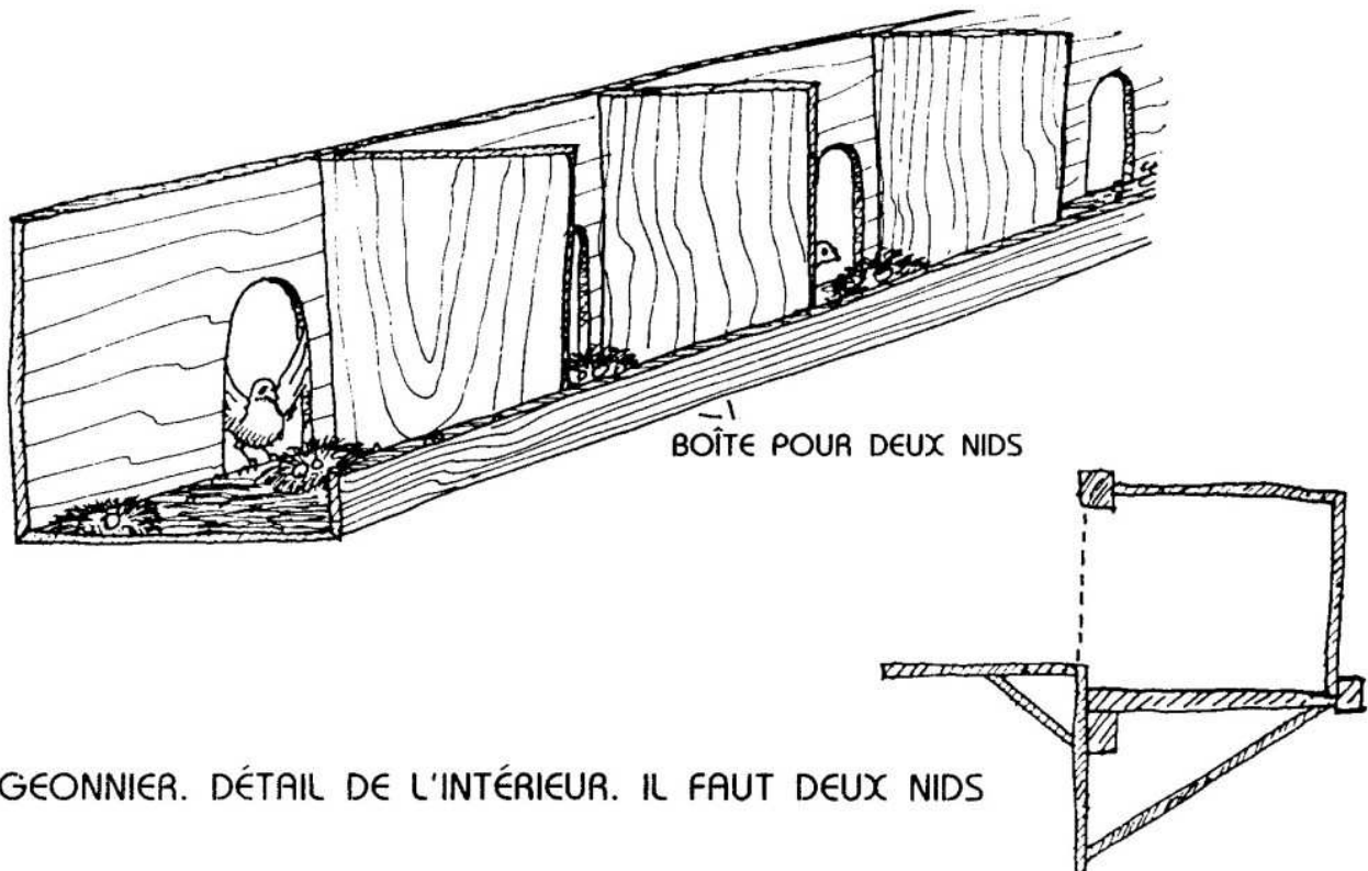
FIG. 5.24: PIGEONNIER. DÉTAIL DE L'INTÉRIER. IL FAUT DEUX NIDS PAR ENTRÉE.
