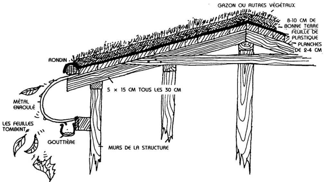
FIG. 6.16: COUPE D'UN TOIT GAZONNÉ.
