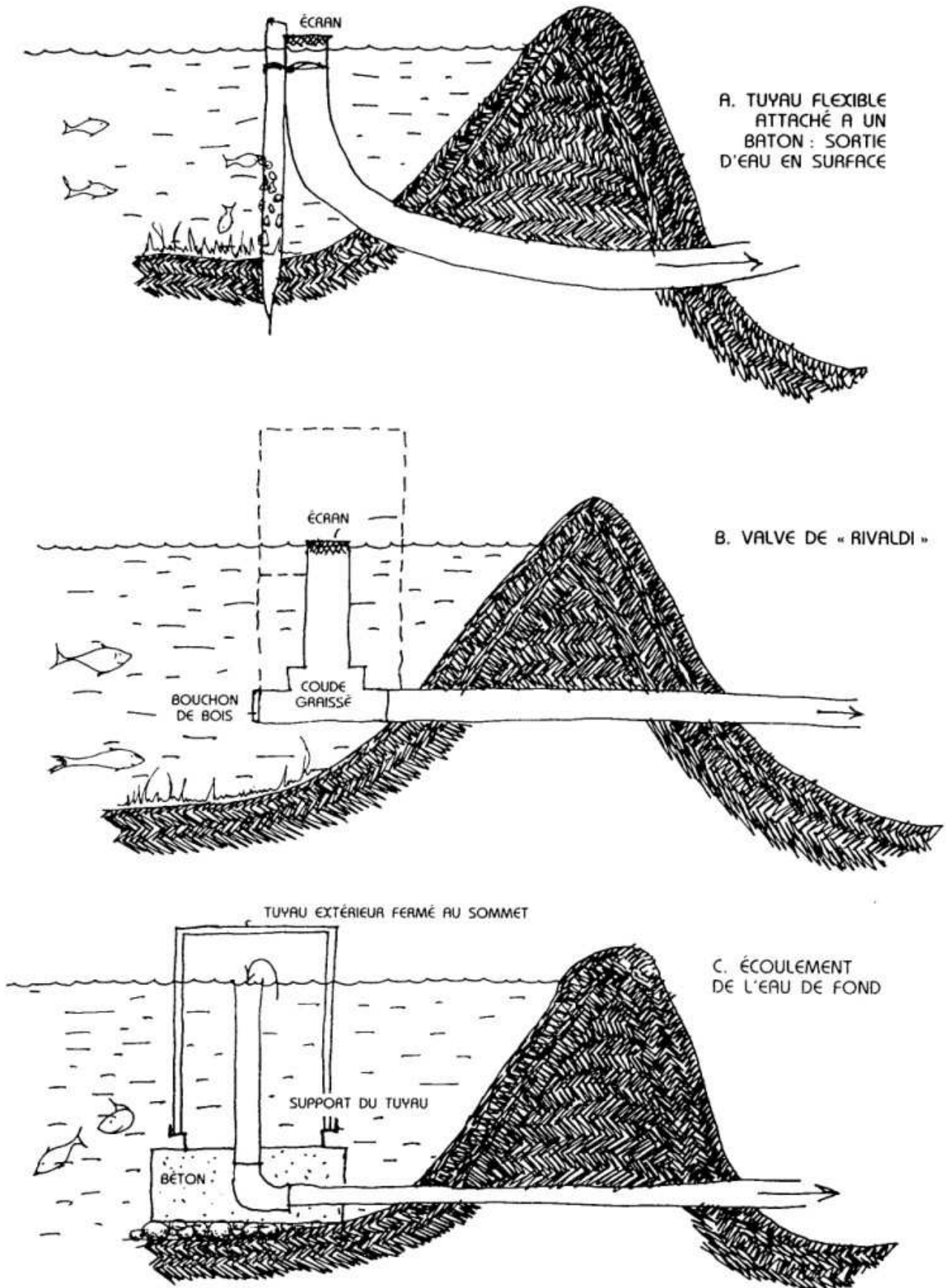
FIG. 7.18 : STRUCTURES DES SORTIES D'EAU DES ETANGS (D'APRES CHAKROFF 16)
