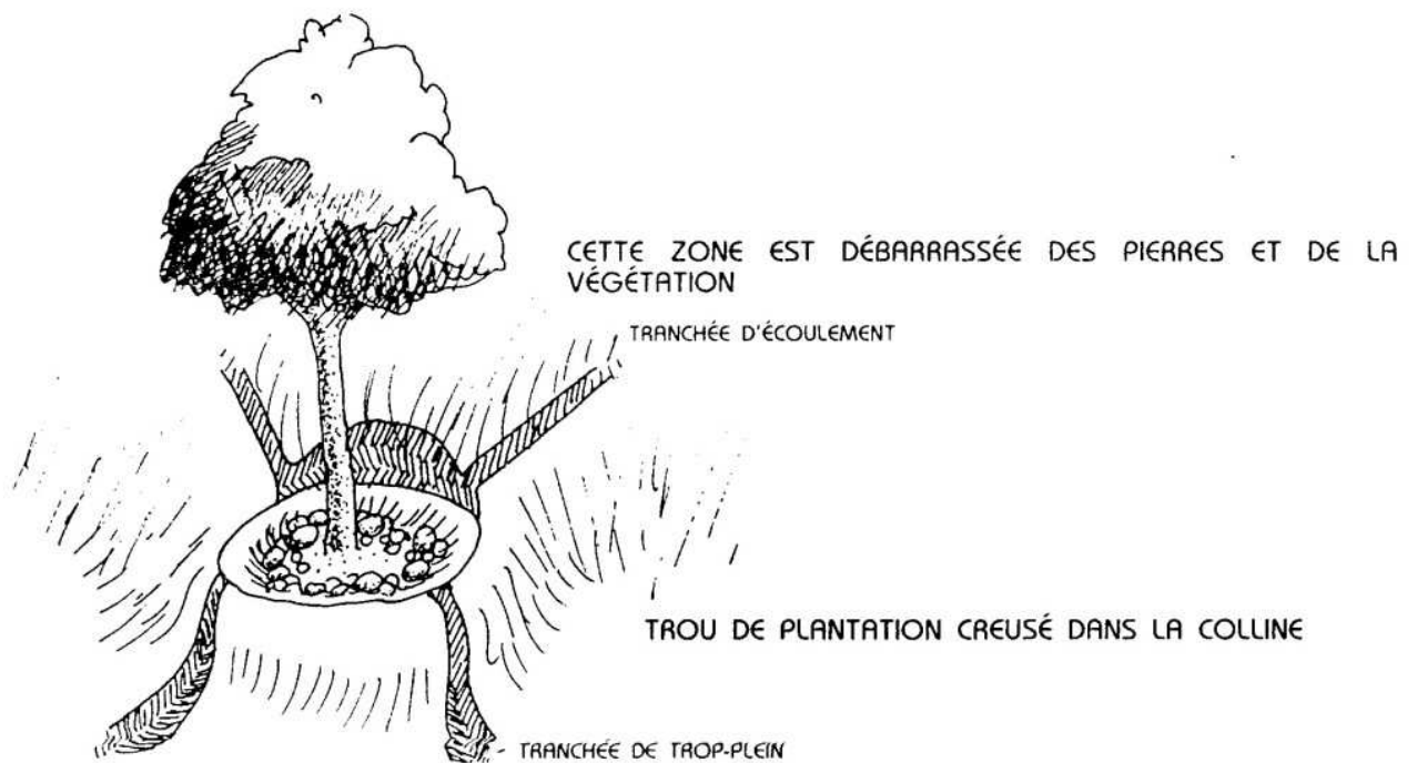
FIG. 5.3 : RÉSEAU ET CUVETTE POUR COLLINE SÈCHE ET PIERREUSE.
