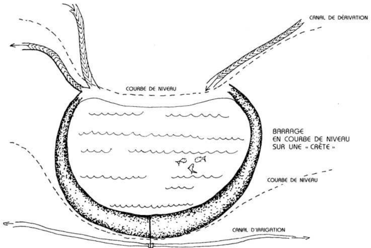
FIG. 7.4 : BARRAGES EN COURBES DE NIVEAU
