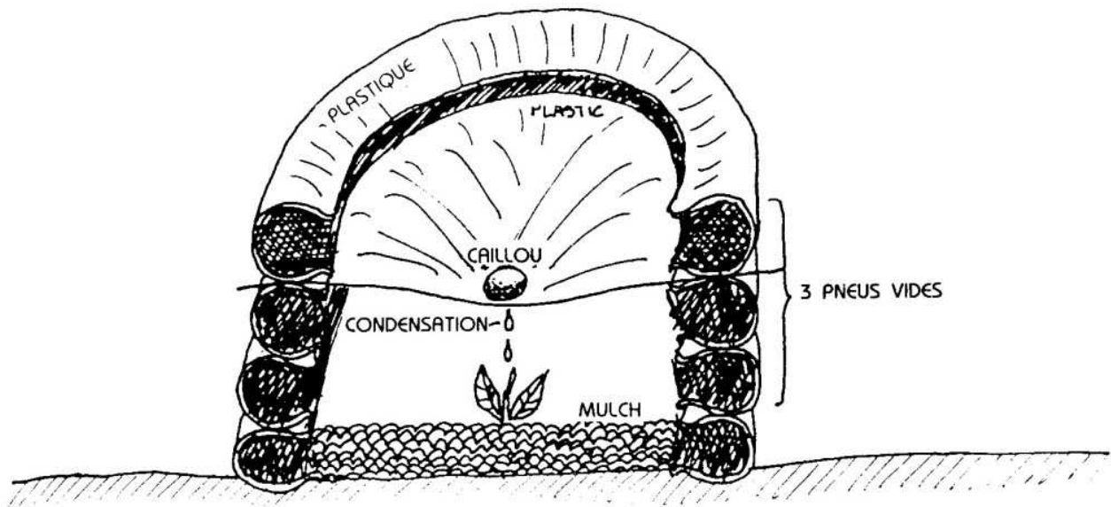
FIG. 5.21 : SERRE EN PNEUS. LE PLASTIQUE CONDENSE L'HUMIDITÉ DE LA NUIT. LA FEUILLE DE PLASTIQUE EST RETIRÉE À LA FIN PRINTEMPS. AUTO-ARROSÉ ET RÉSISTANT AU GEL.
