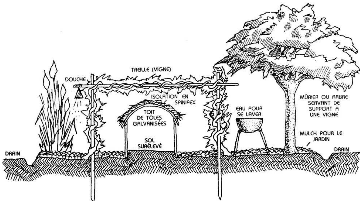
FIG. 5.1 : SECTION D'UNE WILTJA IDÉALE.
