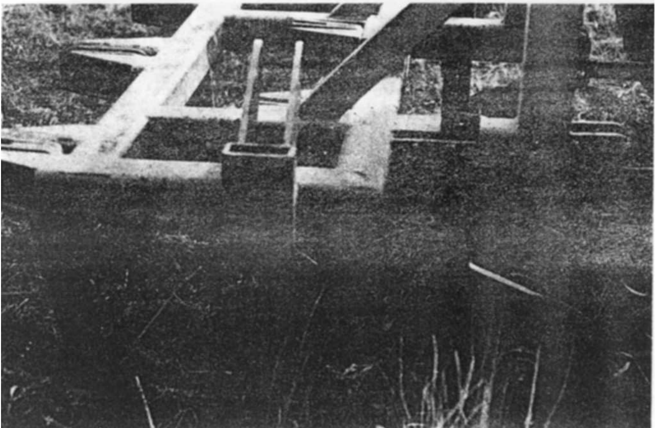
PHOTO 3.2 : DÉTAIL DE LA SOUS-SOLEUSE DE WALLACE. LE COUTRE FEND LE SOL, LES BARRES EMMANCHÉES, EN FOAME DE « SOULIERS SUIVENT, POUR PRATIQUER DES TUNNELS D'AIR SOUS L'HEABE.
