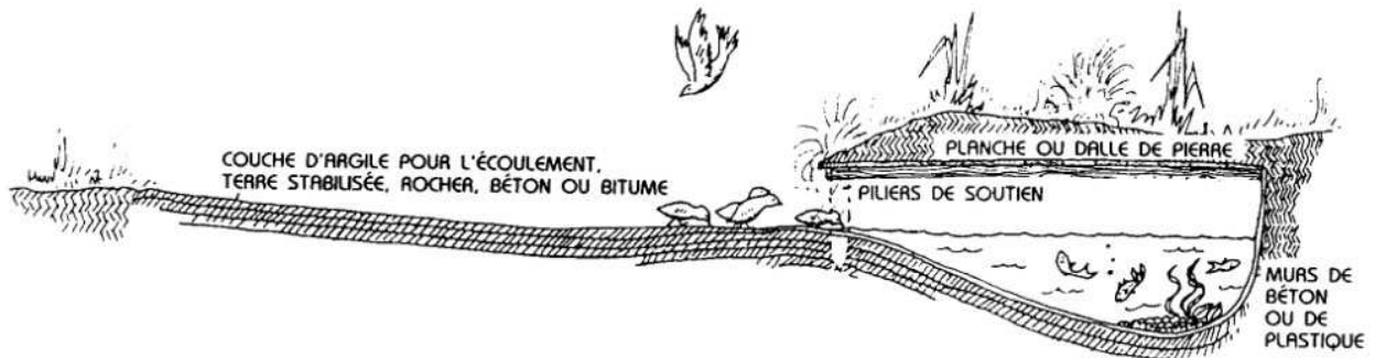
FIG. 5.14: UN PETIT Puits DANS UNE COUCHE D'ARGILE OU A LA BASE D'UN ROCHER RETIENT L'EAU POUR CAILLES, PIGEONS, LÉZARDS ET ABEILLES. POISSONS ET MOULES MAINTIENNENT L'EAU CLAIRE. LE BÉTAIL NE PEUT SALIR DE TELS Puits.
