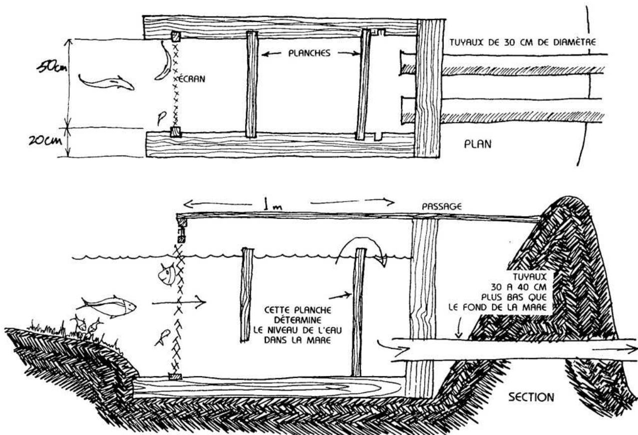
FIG. 7.15: L'ÉCRAN A POISSONS OLASSIQUE « HERGUTH MONK », AVEO TROP-PLEIN POUR ÉCOULEMENT CONSTANT.
