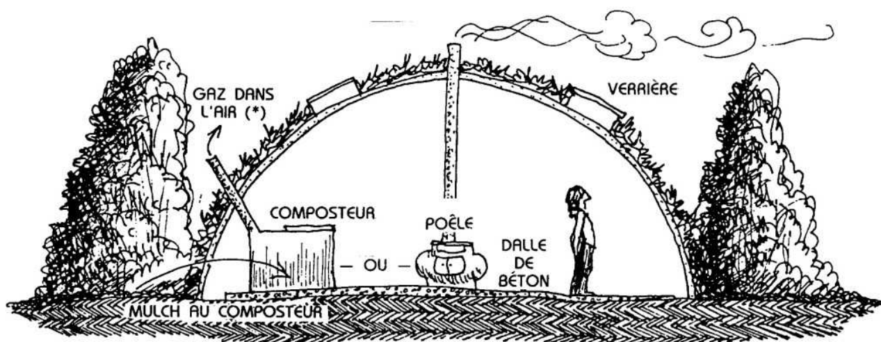
FIG. 6.12: « MAISON DE PLANTES » 3 (SECTION). LE DÔME EST FRIT DE MÉTAL, DE BÉTON, DE PLASTIQUE OU DE BOIS, RECOUVERT DE LIÈRE OU DE GAZON. DES PLANTES ABRITENT LES MURS (D'APRÈS DOERNACH).
