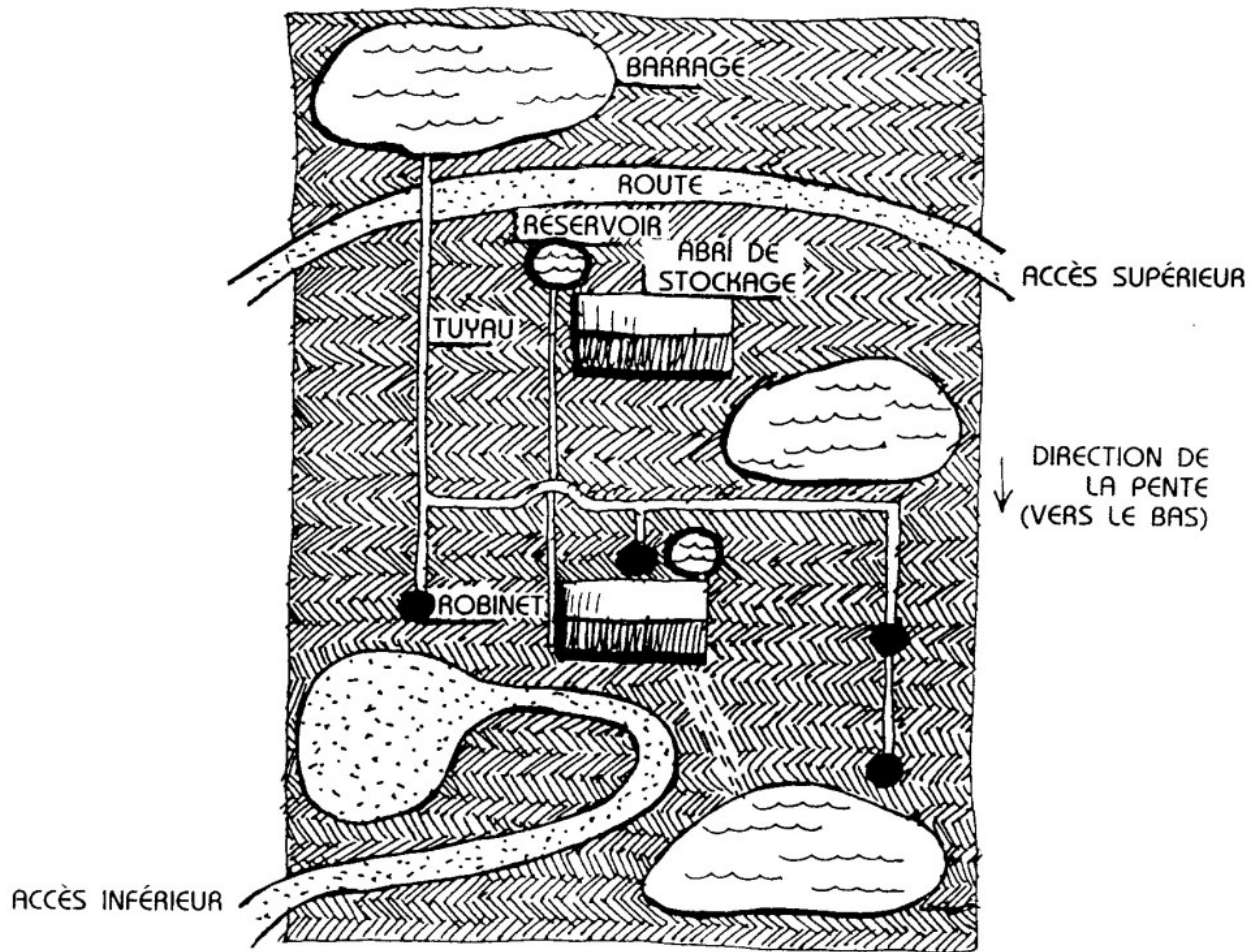
FIG. 210 : PLAN THEORIQUE D'UNE PENTE COMPRENANT EAU ? BATIMENTS ET ACCES
