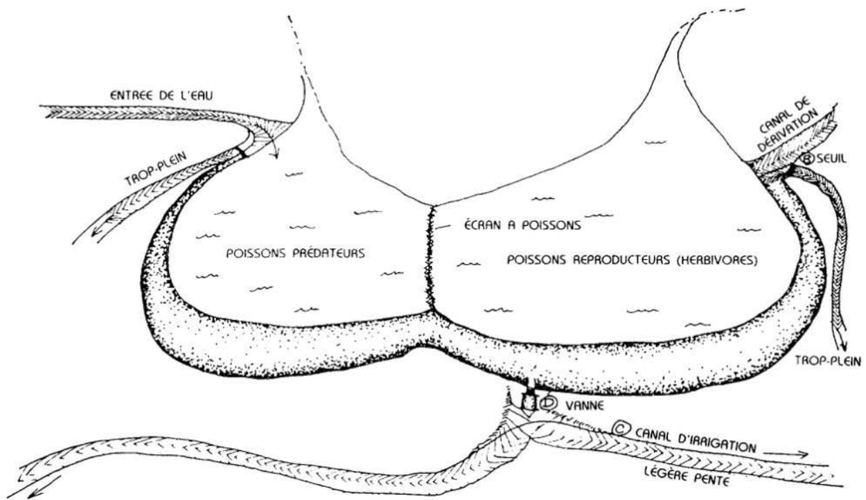
FIG. 7.12: « DOUBLE » BARRAGE DANS UNE DÉPRESSION. LES DEUX PARTIES SONT CONNÉCTÉES PAR UN ÉCRAN A POISSONS. LES PRÉDATEURS (TRUITES) CONTRÔLENT LE NOMBRE DES HERBIVORES (PEACHES) AU MOYEN DE L'ÉCRAN A POISSONS (YANDOIT, VIOTOAIA).
